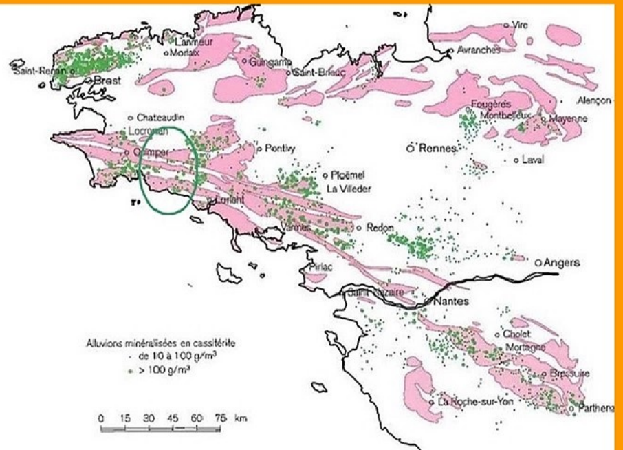
Synthèse de la prospection alluvionnaire pour cassitérite dans le Massif armoricain (d'après Guigues et Devisme, 1969, modifié par Lulzac, 2012). Encart des différents domaines du Massif armoricain d'après Ballèvre et al., 2013.
